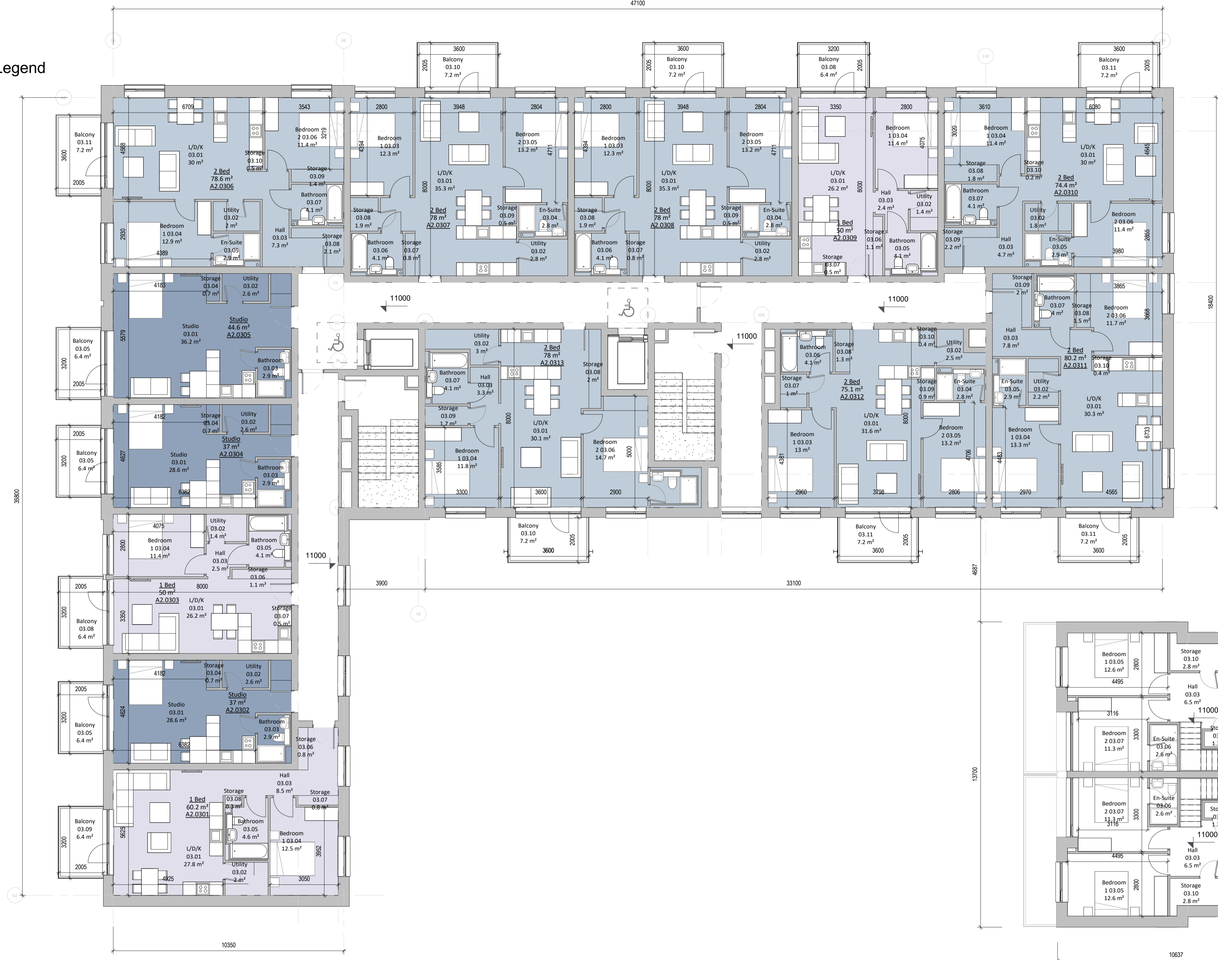
1 A2_03 1:100
